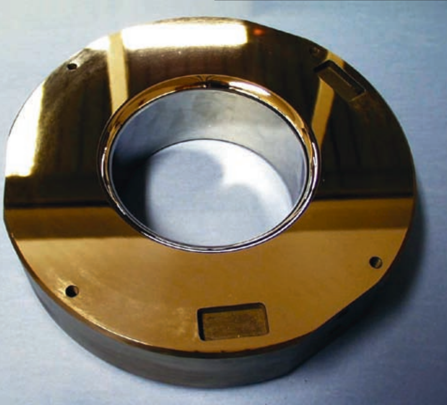
CVD-beschichteter Ziehring, der im oberen Teilbereich nachpoliert wurde
